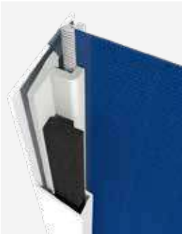
Système pour une meilleure tension de la toile.
