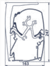
B24 ELITE / PRESTIGE (fixation plafond)
